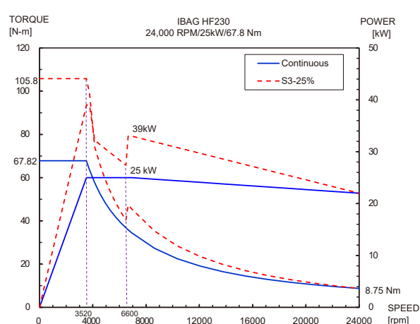
24,000rpm IBAG 內藏式主軸 (選配: H16)
