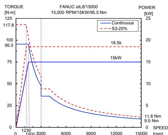
15,000rpm 直結式主軸 (標準: H10,H12E,H16)
