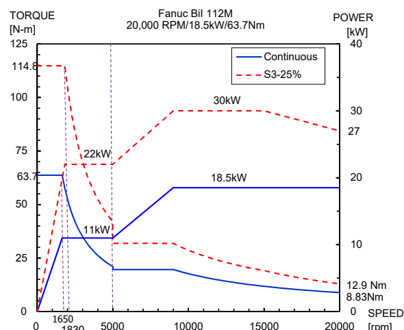
20,000rpm 內藏式主軸 (選配: H10, H12E, H16)
